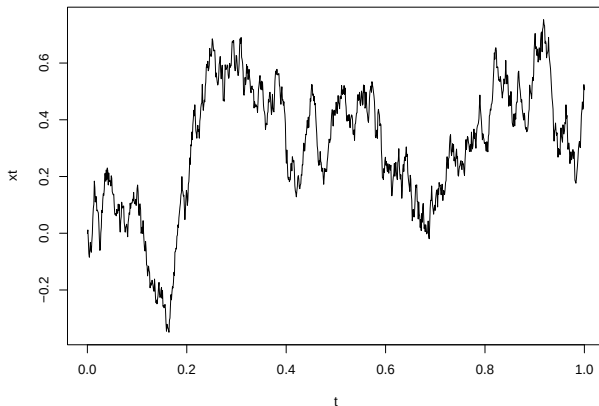
Abbildung 38: Simulierter Wienerprozess, \rho(s, t) = \min(s, t)/\sigma^2
